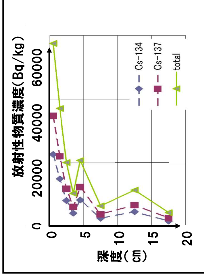
事故前(H23/2月頃)に田起こした田畑の セシウム濃度
