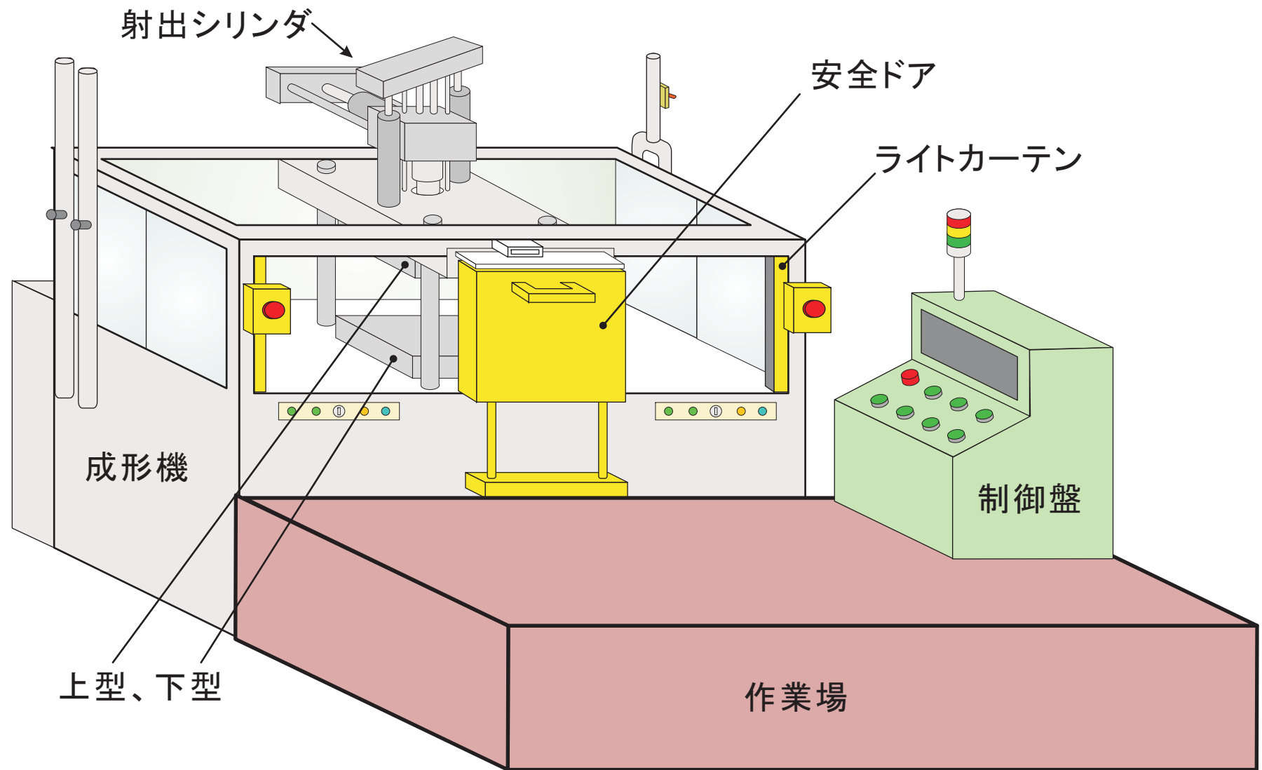
資料2 近接スイッチ成形機の概要図
