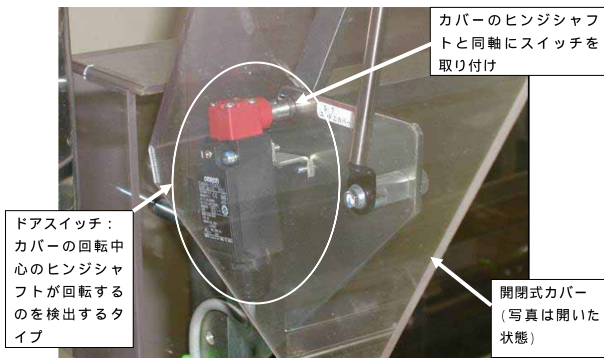
写真2 インターロック付ドアスイッチの採用の例
