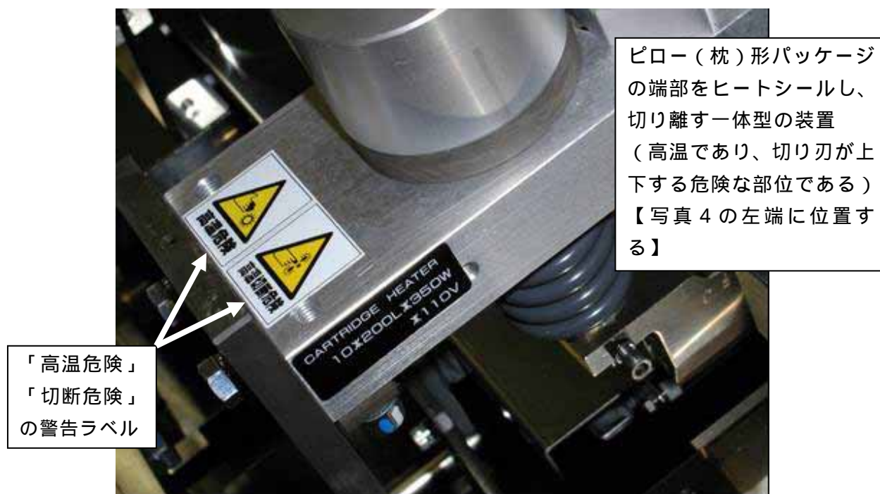
写真3 残留リスク情報（危険部位への警告ラベルの貼付）
