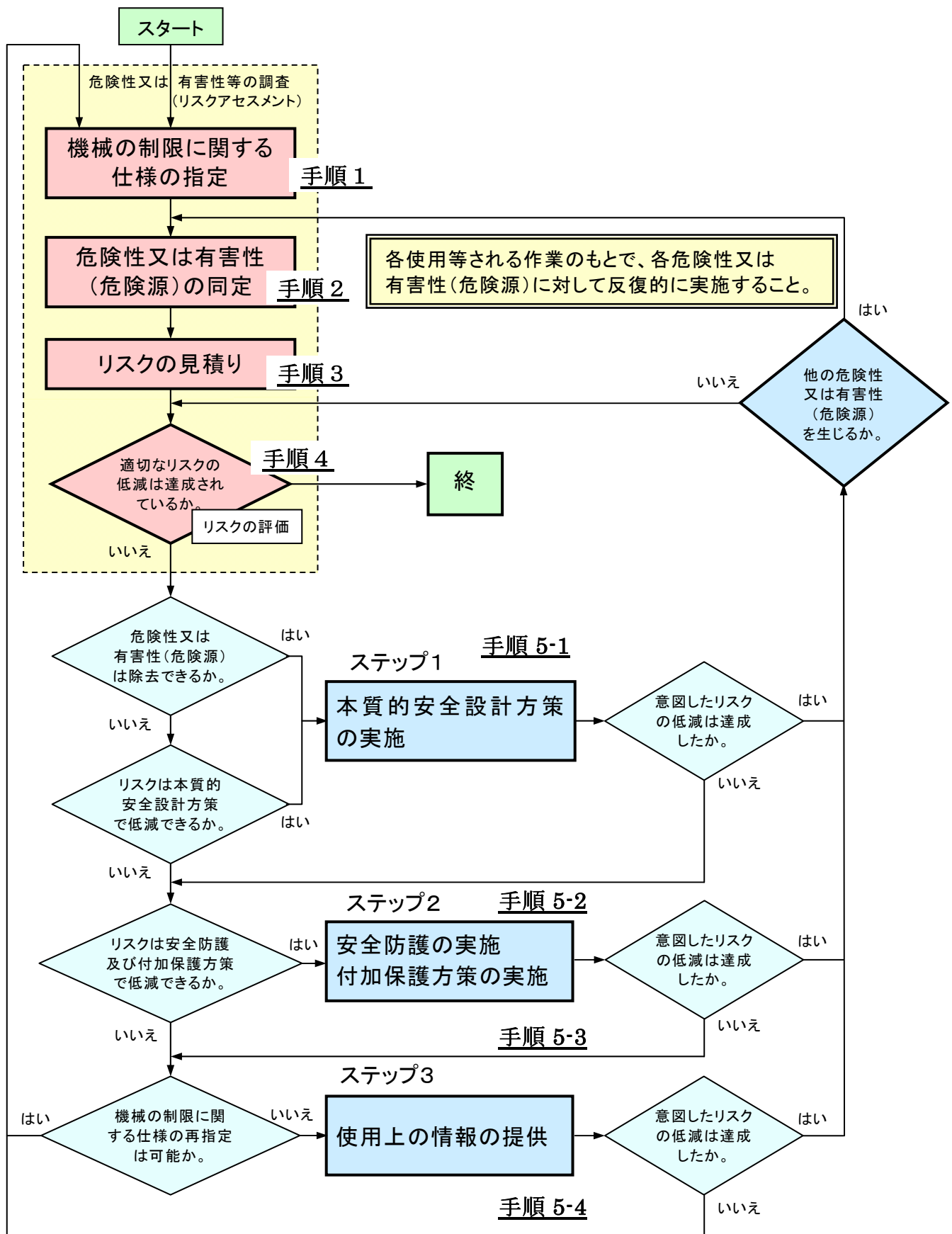
図8 機械の製造等を行う者によるリスクアセスメント及びリスクの低減の手順 (第三章の図8を再録)
