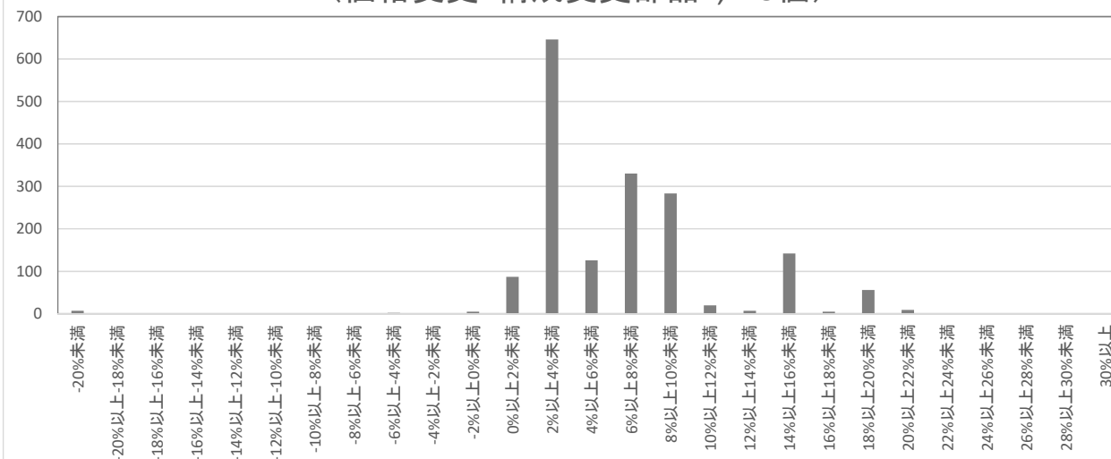
見込利益率の分布 (価格変更・構成変更部品1,279個)
