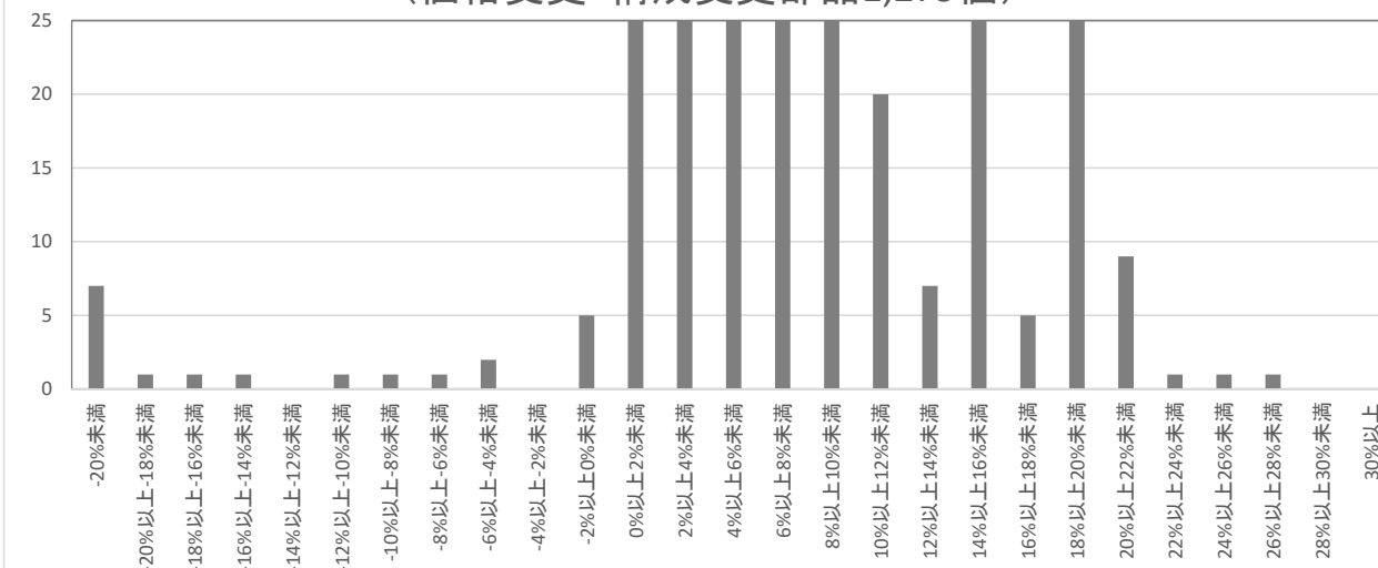
見込利益率の分布(区分件数25件以下のみ拡大) (価格変更・構成変更部品1,279個)
