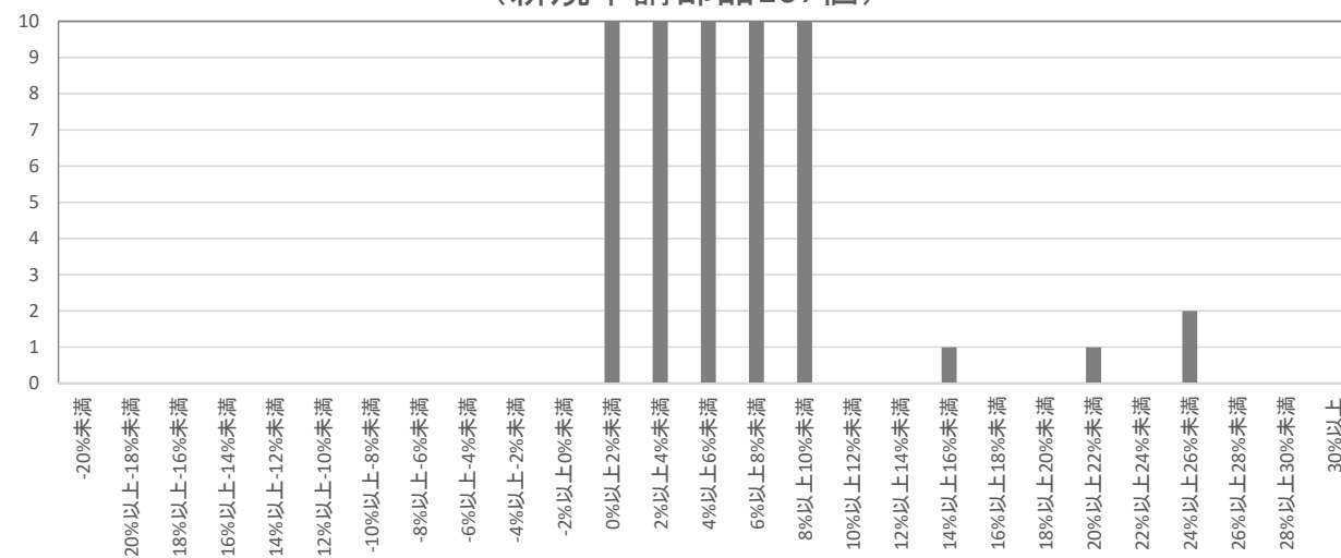
見込利益率の分布(区分件数10件以下のみ拡大) (新規申請部品167個)
