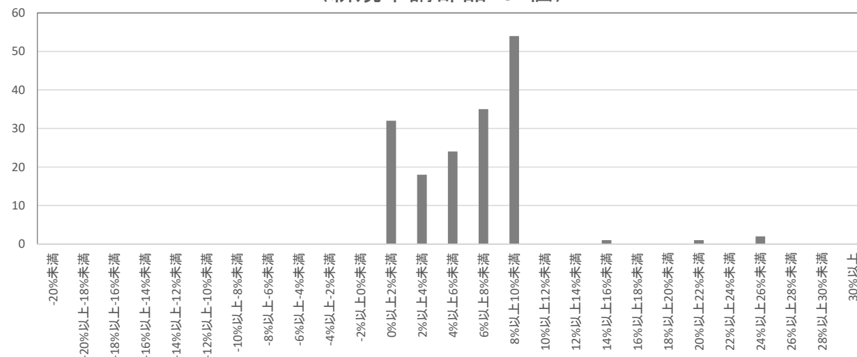
見込利益率の分布 (新規申請部品167個)
