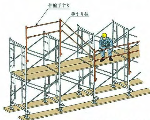
先送り手すり機材の盛替え
