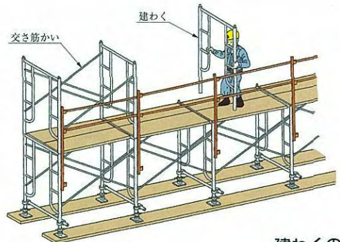
建わくの取付け
