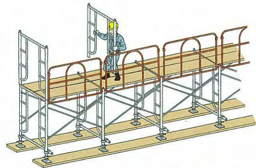
建わくの取付け
