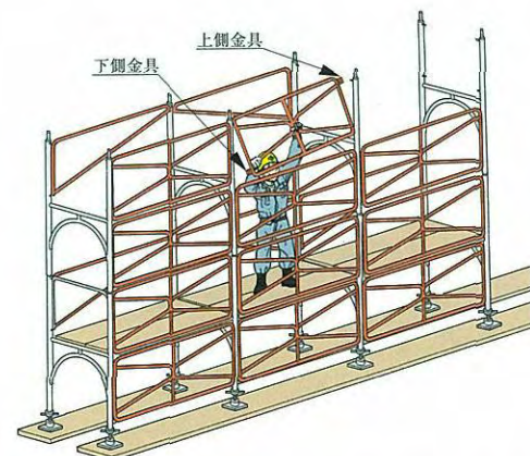
上層の手すり機材の取付け
